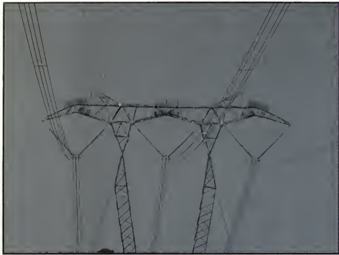
Figure 6: Des “dispositifs de protection des oiseaux en plastique” sont installés sur les tours de transmission pour empêcher les oiseaux de se percher
